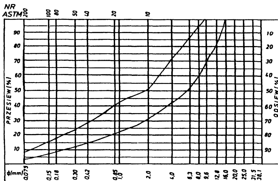
Rys. 9 Krzywe graniczne uziarnienia mieszanki mineralnej 0/16 mm dla warstwy wiążącej, wyrównawczej i wzmacniającej z betonu asfaltowego dla KR 1-2
